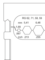
Die profile
