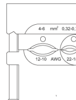
Die profile
