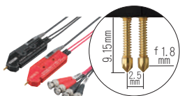
針型探棒L2003 連接線長1.5m
