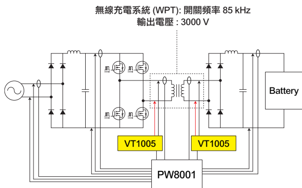
（測量範例）無線充電系統（WPT）的效率測量
